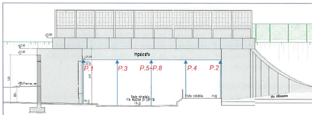
Prospetto frontale
